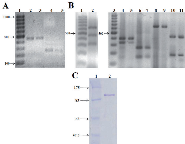
Figura 1. Genes de virulencia expresados por S. pyogenes y E. coli causantes de diarrea. (A) Carril 1: MPM; Carriles 2-3: gen sdaB (440 pb) en las cepas de S. pyogenes SP01 y SP02; Carriles 4-5: gen sdaD (295 pb) en las cepas S. pyogenes SP06 y SP07. (B) Carriles 1 y 3: MPM; Carril 2: genes AA Probe , aggR y aap (629, 457 y 310 pb, respectivamente) de EAEC; Carriles 4-5: genes eaeA y bfpA de EPEC (384 y 324 pb, respectivamente); Carriles 6-7: genes stx2 y stx1 de STEC (255 y 150 pb, respectivamente); Carriles 8-9: gen ial de EIEC (650 pb); Carriles 10-11: genes lt y st de ETEC (450 y 190 pb, respectivamente). (C) Carril 1: MPM; Carril 2: proteína Pic recombinante (109 kDa). Los amplicones mostrados en los carriles 4, 6, 8 y 10 de la figura 2B se obtuvieron con GoTaq® Green Master Mix (Promega®); los demás se amplificaron con Taq ADN polimerasa (Invitrogen®).
