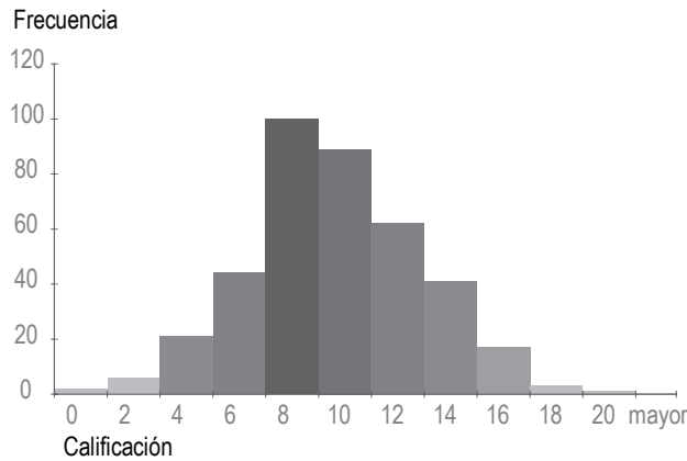
Figura 5. Histograma de Frecuencias para Calificación Global
