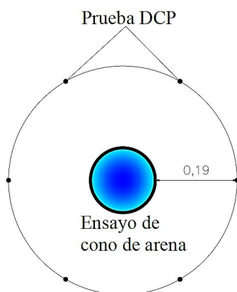
Figura 6. Esquema de pruebas por punto de cono de arena. Fuente: los autores
