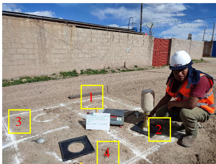
Figura 12. División de la plataforma en 4 sectores y realización del ensayo de CA. Fuente: los autores
