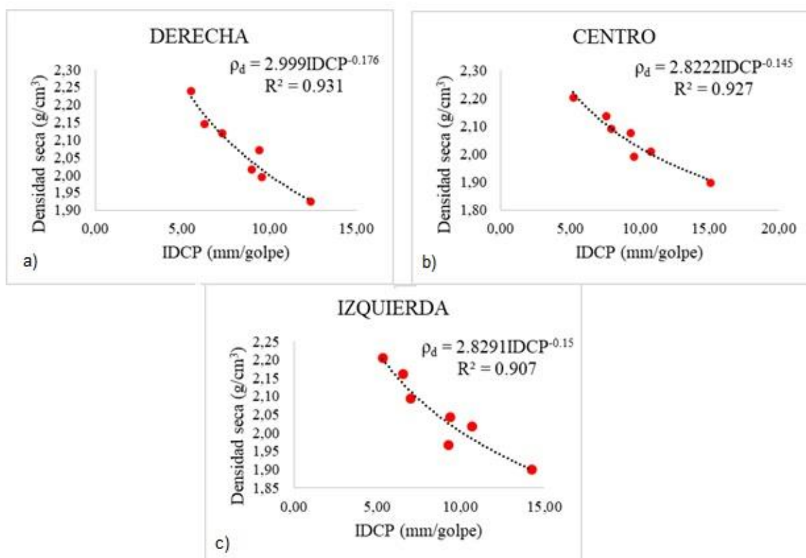
Figura 9. Variación del IDCP vs \rho_d en la franja derecha. Fuente: los autores
