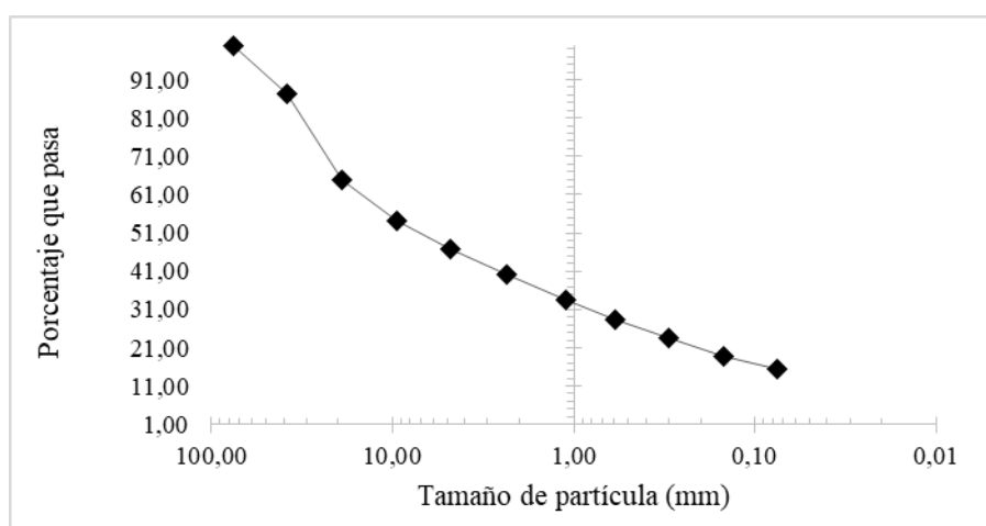
Figura 3. Curva granulométrica de la muestra. Fuente: los autores
