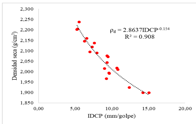
Figura 8. Variación del IDCP vs \rho_d . Fuente: los autores
