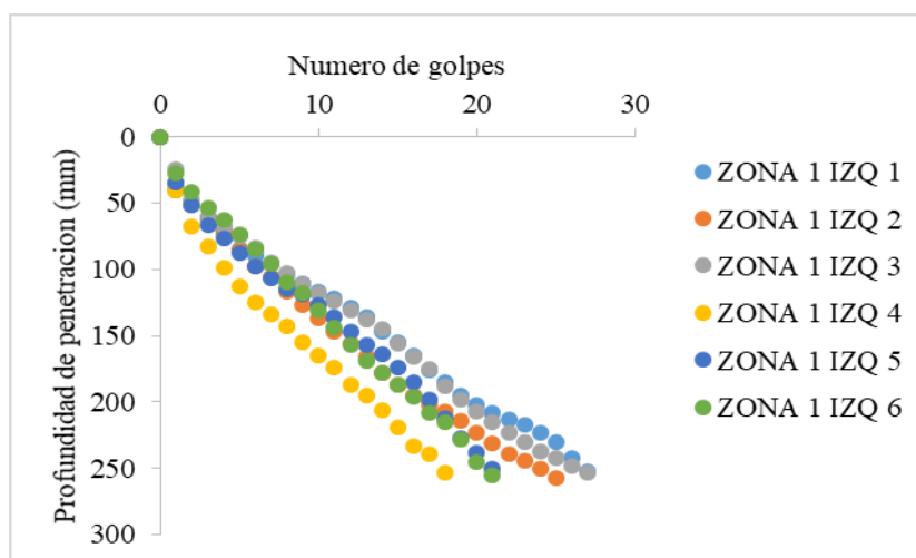
Figura 10. Curva DCP vs golpes acumulados de la zona 1. Fuente: los autores
