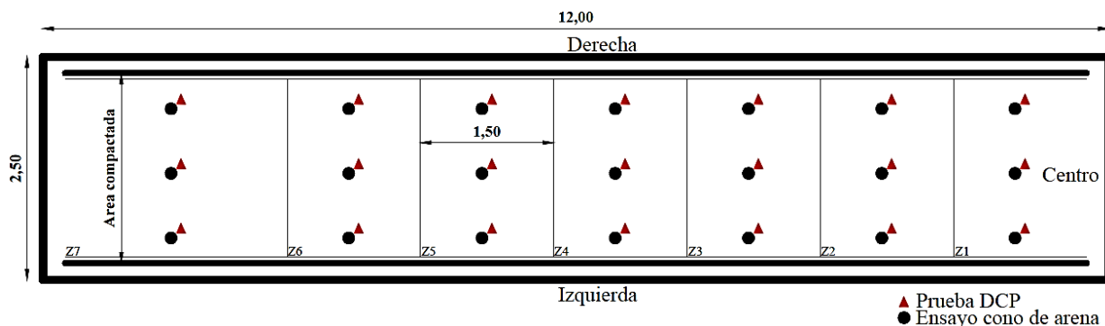
Figura 5. Esquema de relleno de pruebas. Fuente: los autores
