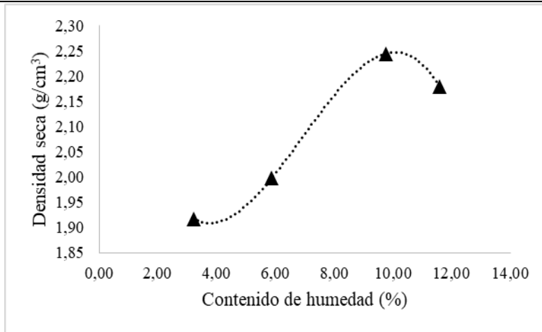
Figura 4. Curva de compactación (Proctor modificado). Fuente: los autores
