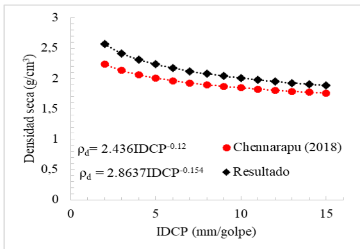
Figura 11. Comparación de IDCP vs \rho_d del presente estudio el de [1]. Fuente: los autores
