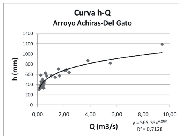
Figura 10. Curva de gastos del arroyo Achiras-del Gato en sección Ruta 8
