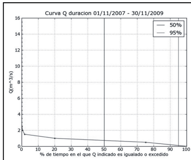
Figura 16. Curva Qd nov2007-2009 (post-presa)
