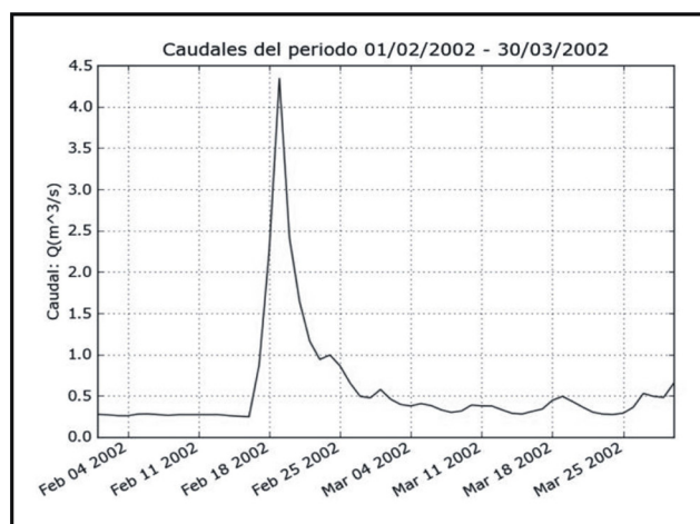
Figura 13. Hidrograma feb-mar 2002
