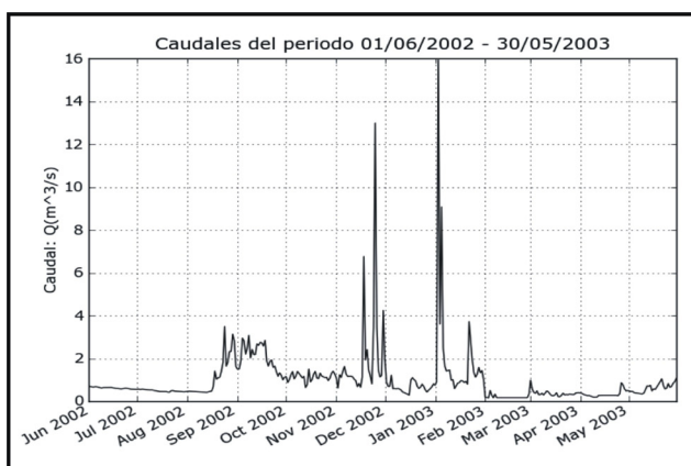
Figura 12. Hidrograma jun 02-may03
