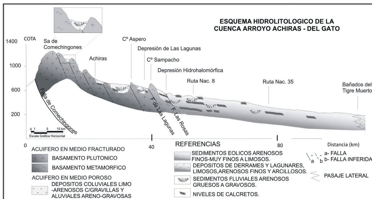
Figura 4. Hidrolitología en la cuenca del arroyo Achiras-del Gato. (Fuente: Degiovanni et al. 2005)
