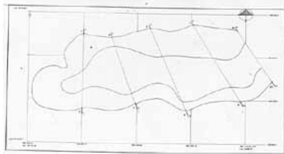
Figura 3. Vista en planta y ubicación de las secciones transversales en las Cárcava
