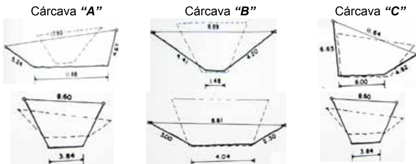
Figura 4. Secciones Transversales de las Cárcavas
