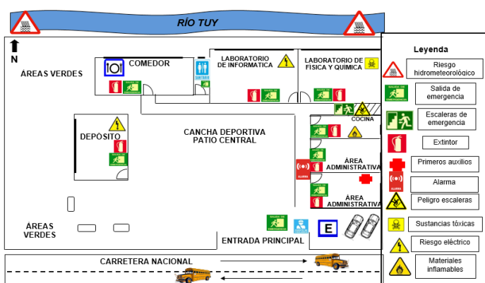
Gráfico 1c. Plano de riesgos y rutas de escape para la atención de amenazas hidrometeorológicas en la U.E.N. "Liceo Bolivariano Panaquire". Nivel PB.
