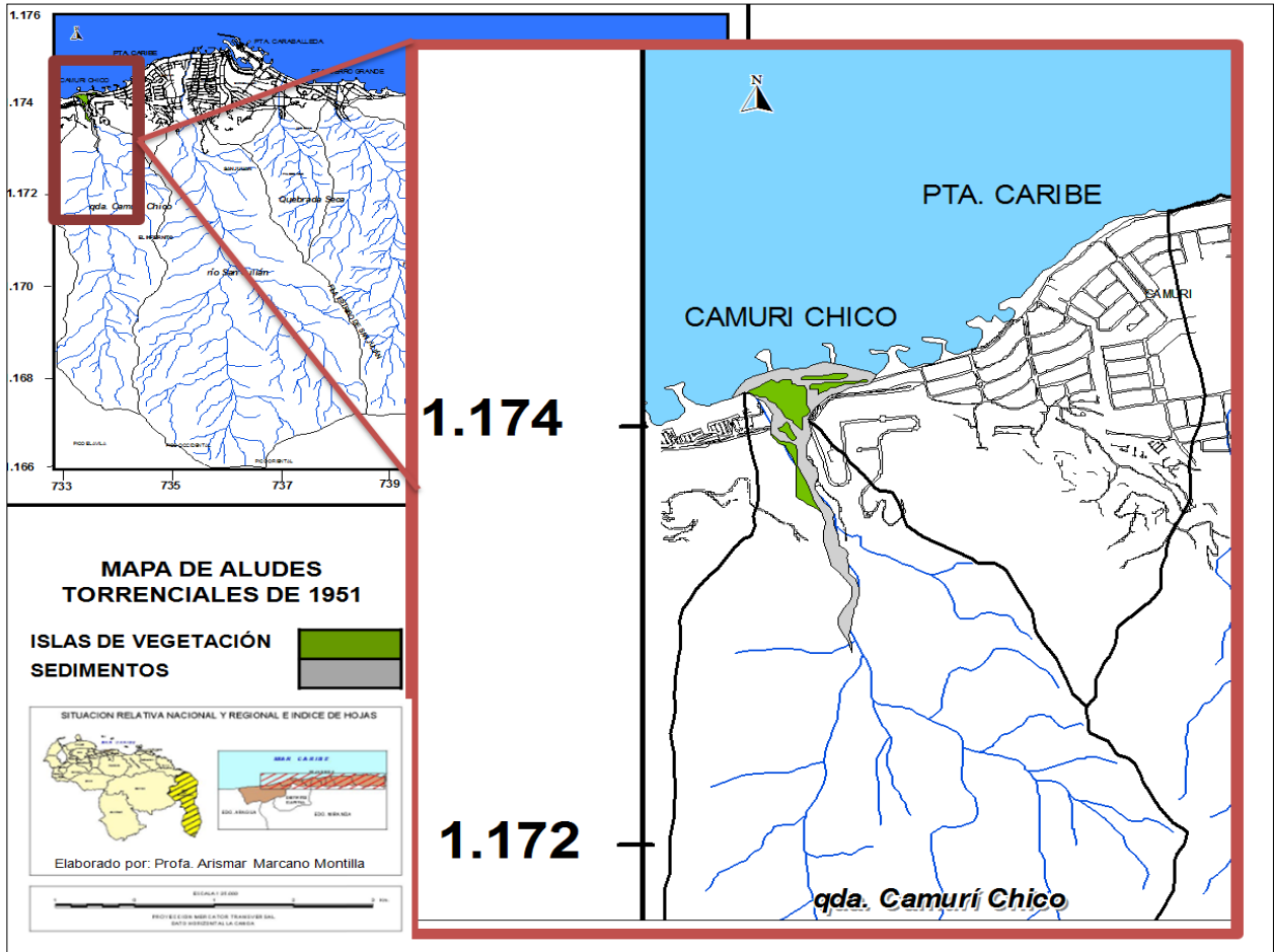
Gráfico 3. Mapa de aludes torrenciales de 1951. Tomado y modificado de “Proyecto Ávila: Mapa de Riesgo” a escala 1:25.000 por IGVS/MARN, 2002, Caracas.
