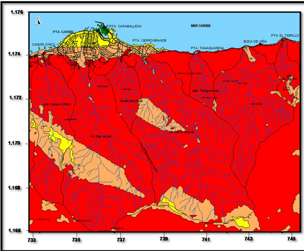
MAPA DE AMENAZAS A LOS MOVIMIENTOS EN MASA CONSIDERANDO LA SISMICIDAD COMO DESENCADENANTE
