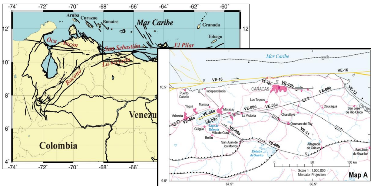
Gráfico 1. Mapa de fallas principales de la región centro-norte de Venezuela según Beltrán. Tomado de "Mapas de Fallas Cuaternarias de Venezuela" a escala 1:2.000.000 por R. Vásquez, 2000, Caracas.
