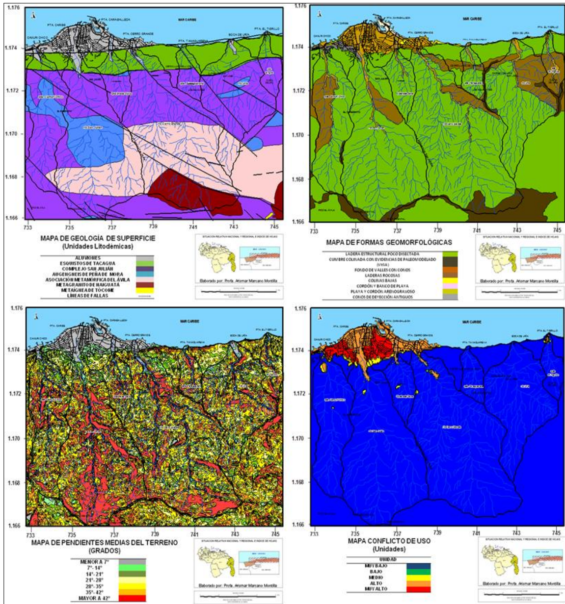
Gráfico 7. Mapas básicos considerando las variables: Geología de superficie, geomorfología, pendiente media del terreno y conflicto de uso. Generados por el SIG a partir del “Proyecto Ávila: Mapa de Riesgo” a escala 1:25.000 por IGVS/MARN, 2002, Caracas y el MDT. Georeferenciada con la proyección cartográfica UTM-SAD69, Uso Horario 19, Hemisferio Nor.
