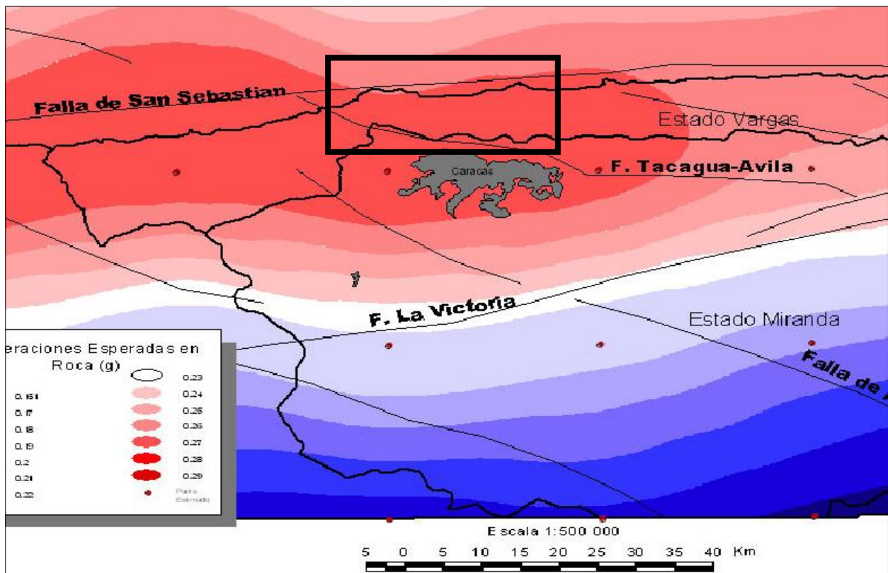
Gráfico 2. Evaluación de la amenaza sísmica, aceleraciones esperadas en roca. Tomado de “Síntesis de la nomenclatura de la unidades de rocas ígneas y metamórficas de la Cordillera de la Costa, Venezuela” por F. Urbani, 2005, Instituto de Materiales y Modelos Estructurales (IMME) , 42 (2).
