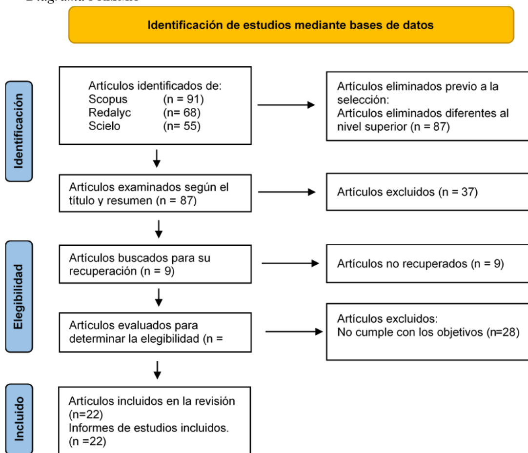
Figura 1 Diagrama PRISMA
