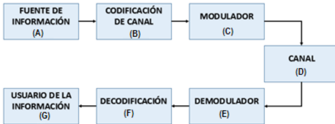
Figura 1. Diagrama de bloques simplificado del sistema de comunicaciones con codificación Reed-Solomon modelado en LabVIEW
