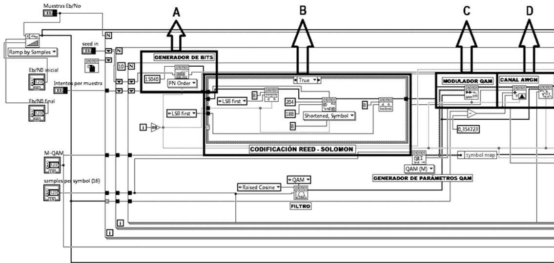
Figura 2. Principales etapas en transmisión del modelo de sistema de comunicaciones con codificación
